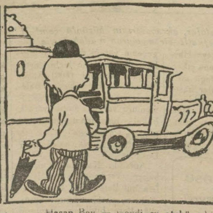
3: Hasan Bey — Naydi şu otobüse binip "Çekirge" den Bursaya gidelim.
